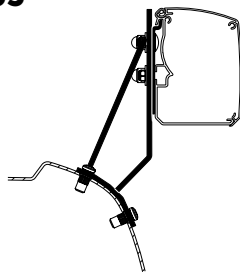
Kit staffe Thule 3200 VW Transporter 2025 e Ford Custom V710
