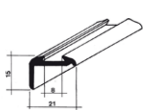
41214.AA Riloga Lamiera-tetto/parete
