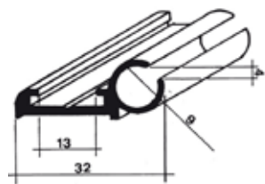
41215.AA Riloga Portaveranda
