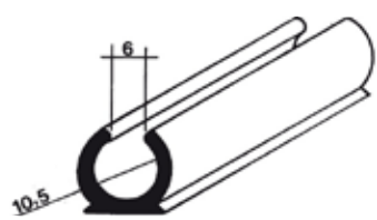
41217.AA Profilo Portaveranda-oscuranti
